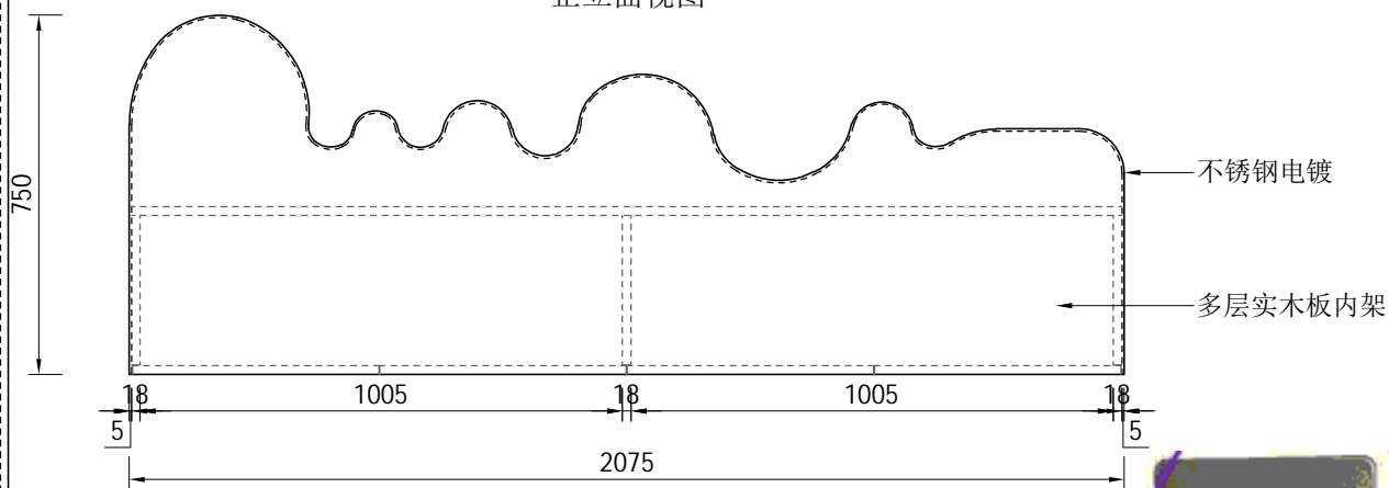
① Plan 平面图
