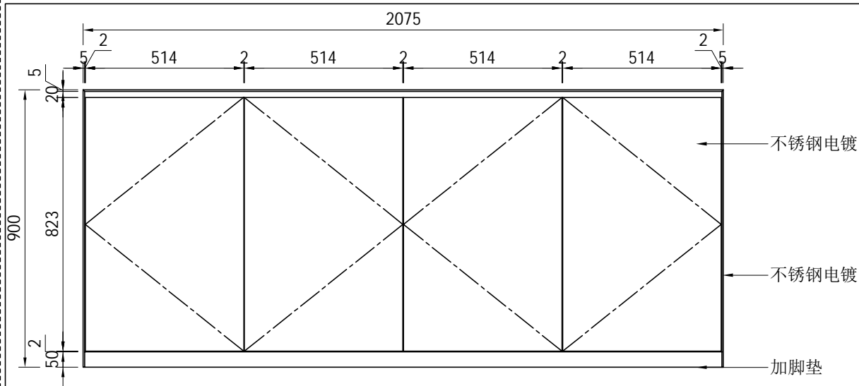
② Elevation 正立面视图
